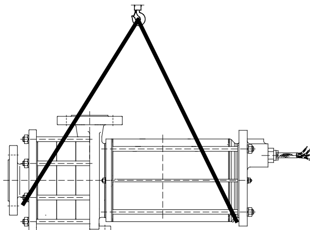
Rys. 5: Przymocowanie podnośnika do agregatu pompy
