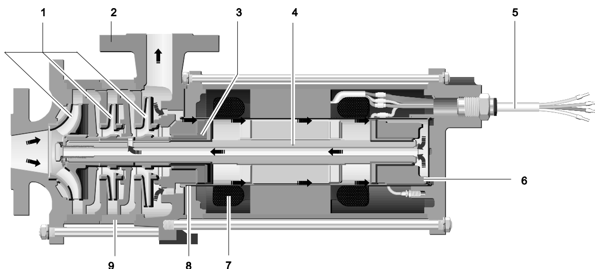
Rys. 4: Budowa CAM (przykład CAM 2/3)
