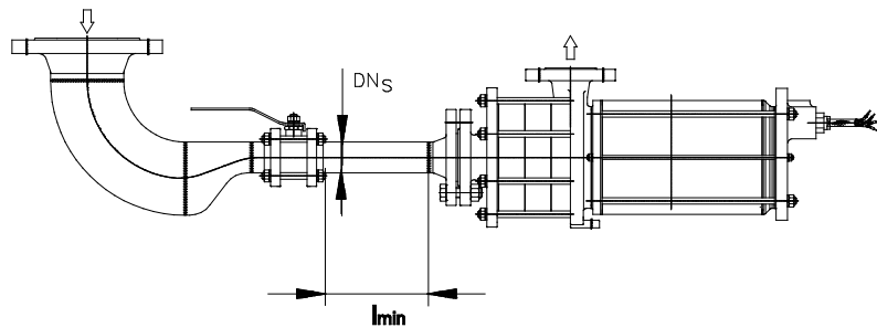
Abb. 7: Zulaufleitung
