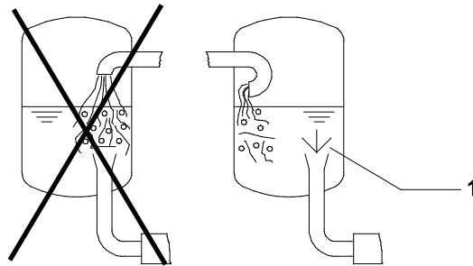
Abb. 9: Anordnung Tankeinlauf/Tankauslauf
