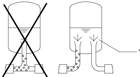
Abb. 11: Anordnung Parallelbetrieb
