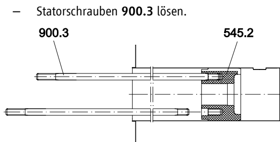
Abb. 14: Demontage des Kohlelagers
