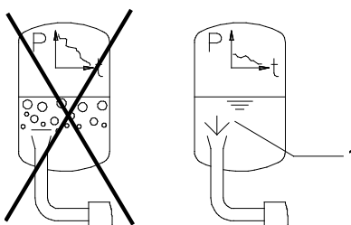
Abb. 12: Langsame Druck-/Temperaturabsenkung
