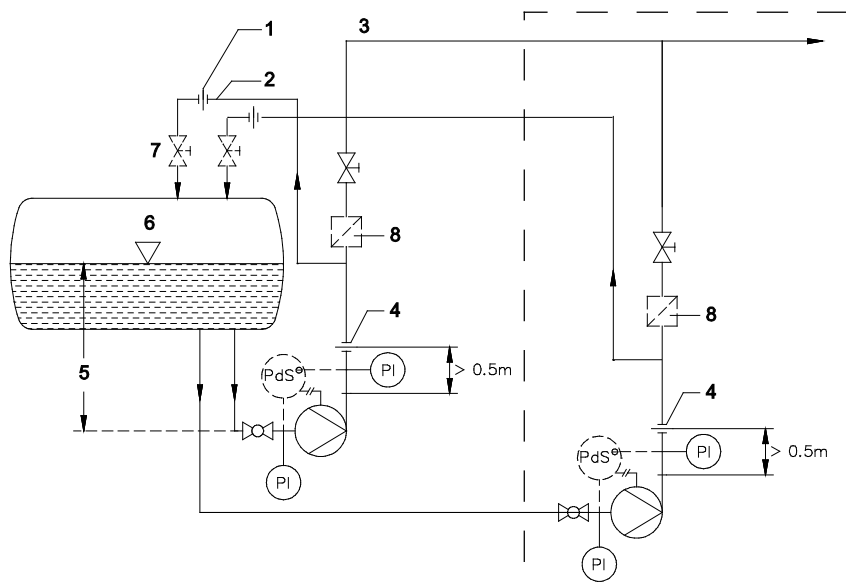
Abb. 13: Automatische Entgasung (Einzelpumpe-Parallelpumpen)
