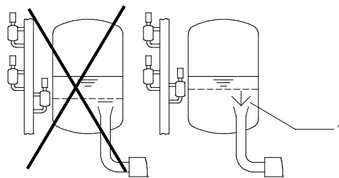
Abb. 10: Anordnung Niveauüberwachung
